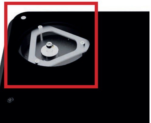
Abb. 10: Einstellung des Anti-Skating
