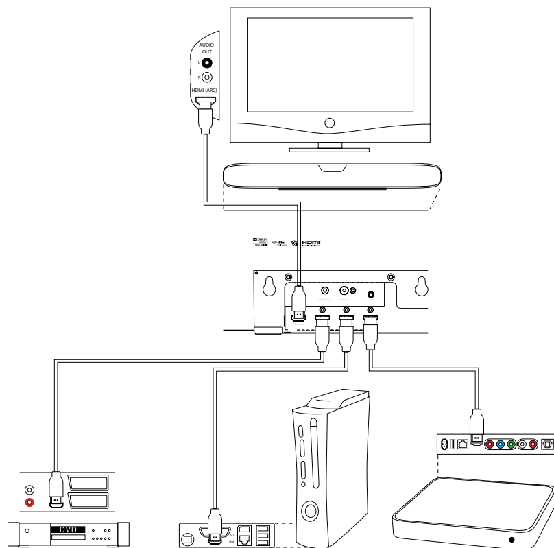
Afbeelding 4 De Panorama 2 aangesloten op een home-entertainmentsysteem
