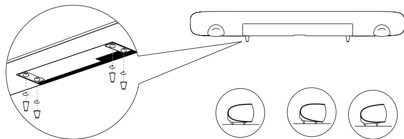
Figur 2 Montering av fötter
