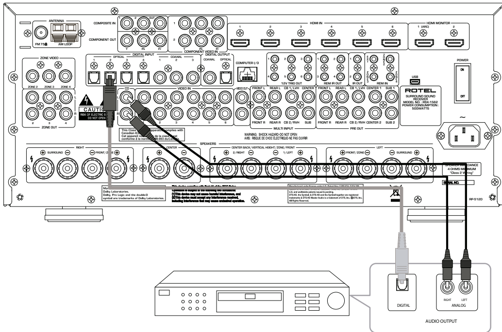
Рис. 8: Подключения CD-плеера
