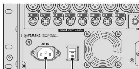
Переключатель питания Разъем AC IN
